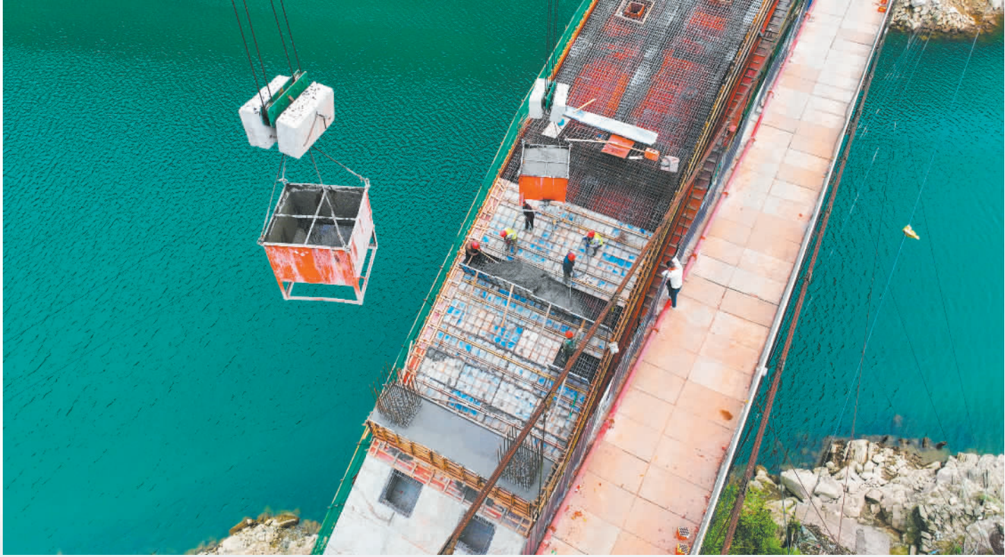
►4月11日,重庆市酉阳土家 族苗族自治县龚滩镇跨江渡改桥施 工现场。该桥建成后,将便利阿蓬 江两岸村民出行。 邱洪斌摄(中经视觉)
