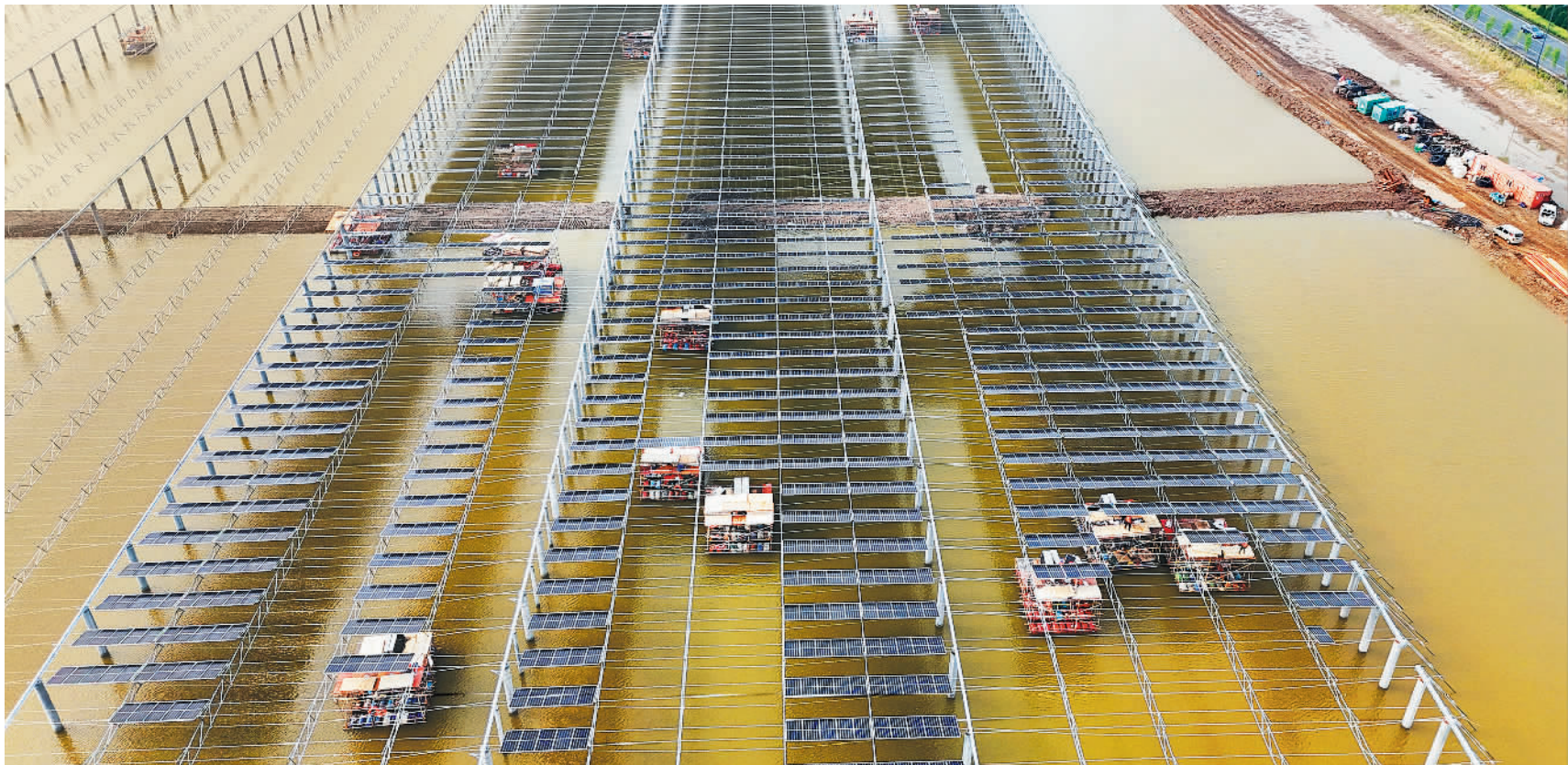
4月22日，江苏省连云港市三峡青口盐场渔光互补光伏复合项目建设现场，工人正加紧施工。该项目总投资约20亿元，将光伏电站与水产养殖融合，构建绿色生态循环体系。
