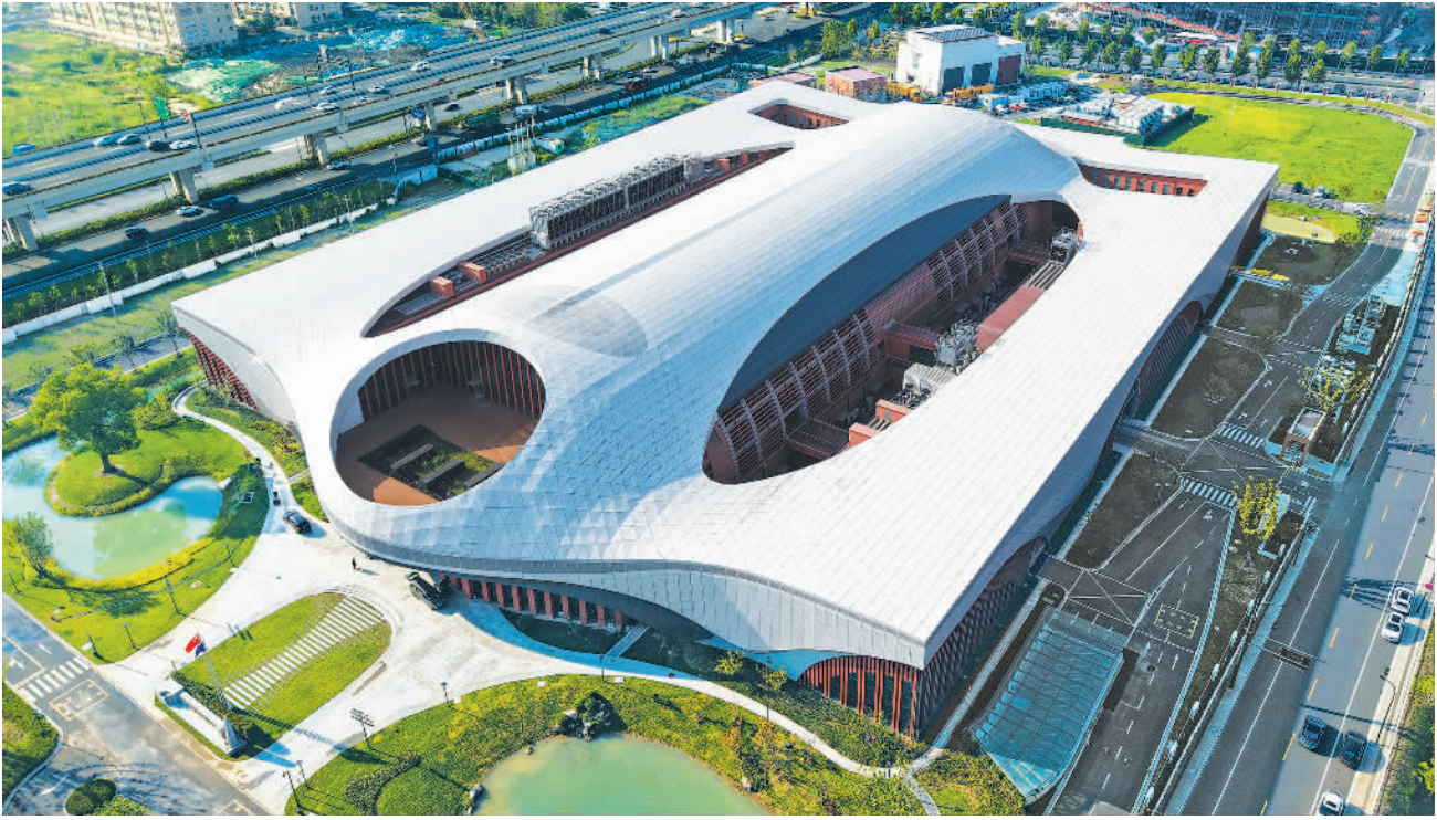
9月29日,位于浙江杭州的国家重大科技基础设施——浙大超重力离心模拟与实验装置的核心设备正式启用。据了解,这套由我国完全自主研发的超重力大科学装置,能以很小的尺寸、极短的时间再现真实世界的变迁,为推演验证千米尺度灾变、万年历时污染迁移等提供关键支撑。图为浙大超重力离心模拟与实验装置实验大楼。
